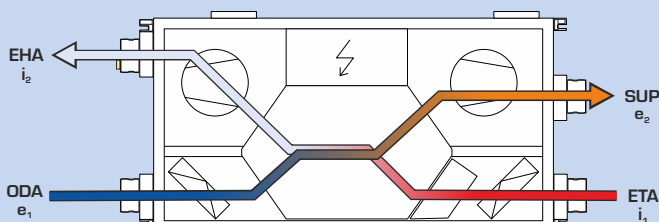
1. rovnotlaké větrání s rekuperací tepla
