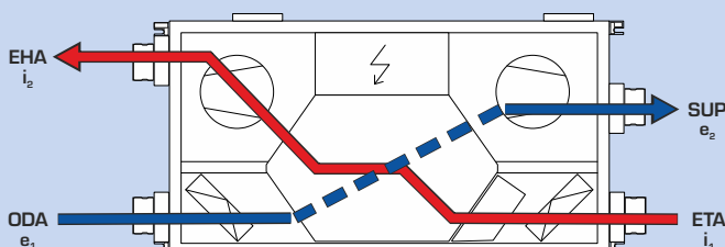
2. noční vychlazování by-passem v létě
